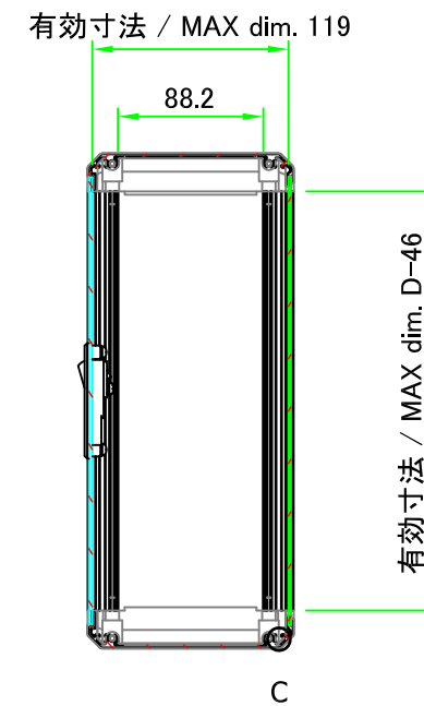
B-B ( 1 : 5 )
